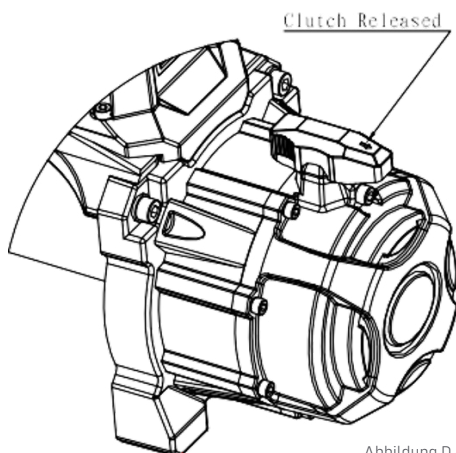
Abbildung D - Ausgelöste Kupplung
