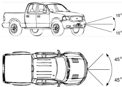
Abbildung H - Maximale Windenwinkel der Rollenklüsen
